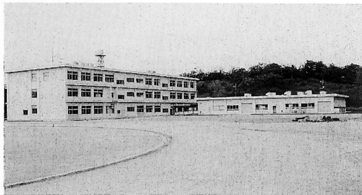
工 業 棟
